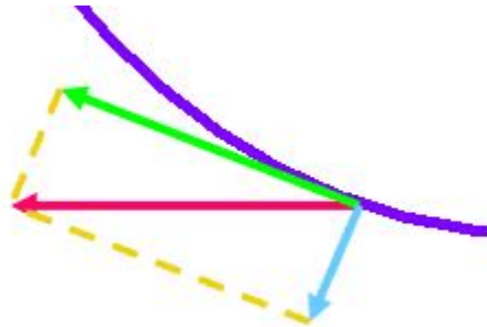
El campo F (en rojo) y su componente tangencial (en verde).
