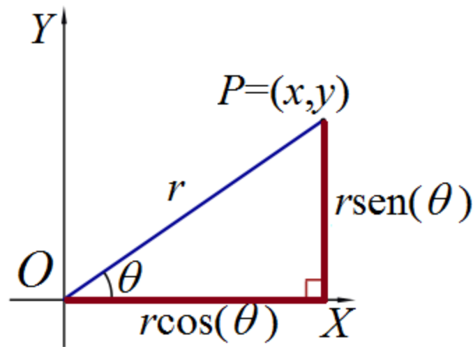
Coordenadas polares y cartesianas.
