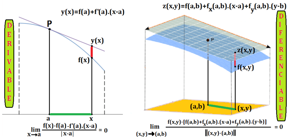
Derivabilidad (1D) frente a diferenciabilidad (2D)
