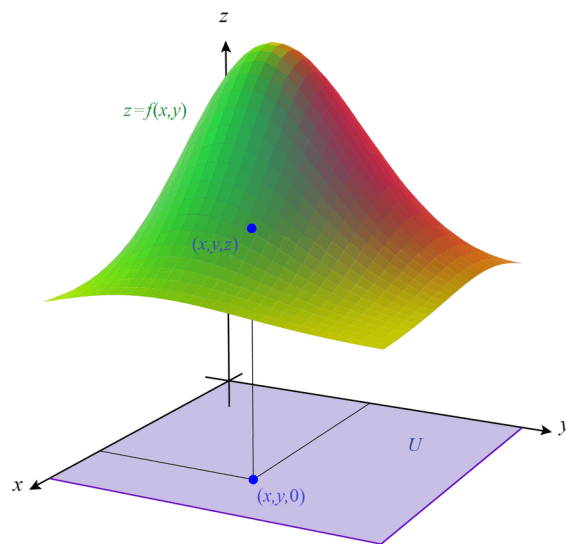
Superficie de ecuación z = f(x, y) .
