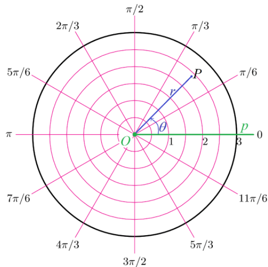
Coordenadas polares.
