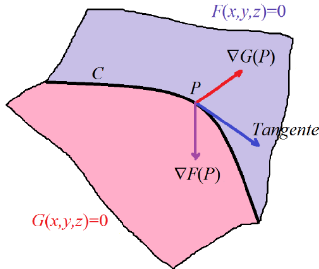
Curva dada por ecuaciones implícitas.
