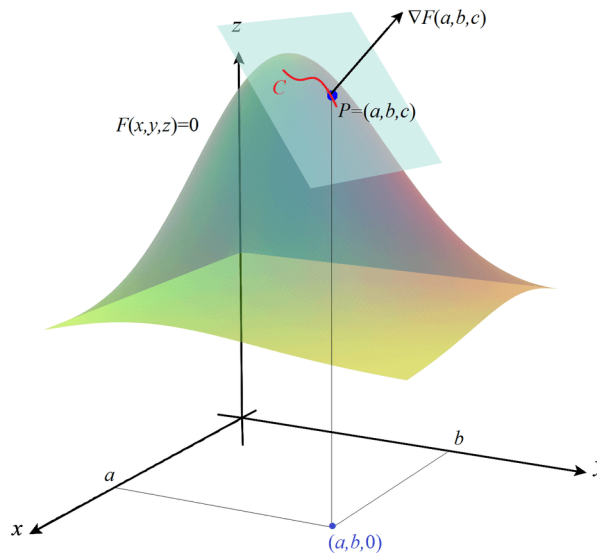
Normalidad del diferencial y plano tangente.
