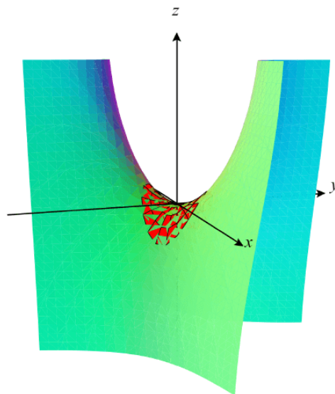
La superficie z + \sin(z) + x^2 + y^2 - 6xy = 0 y la gráfica del polinomio de Taylor p_2(x, y) .
