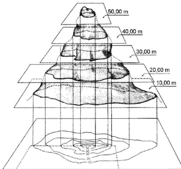
Curvas de nivel para c = 10, 20, \dots, 50 metros.
