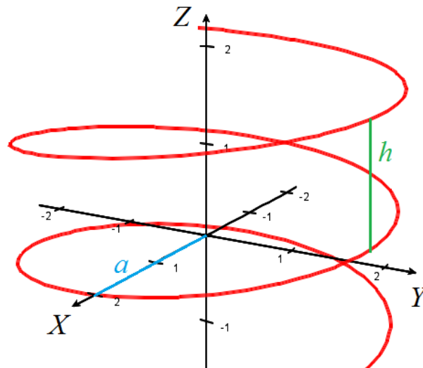
Hélice circular recta.
