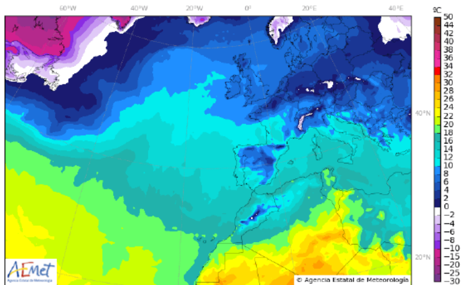
Isotermas.
