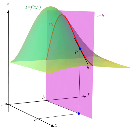
Interpretaciones geométricas de \frac{\partial f}{\partial x} (izquierda) y de \frac{\partial f}{\partial y} (derecha).
