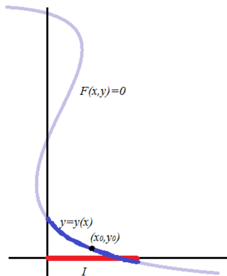
Interpretación geométrica del teorema de la función implícita.
