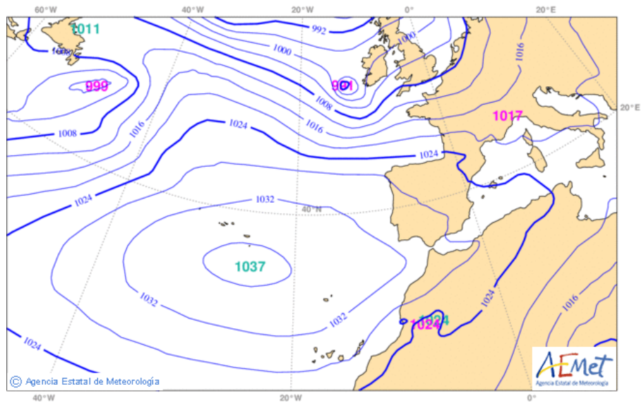
Isobaras.
