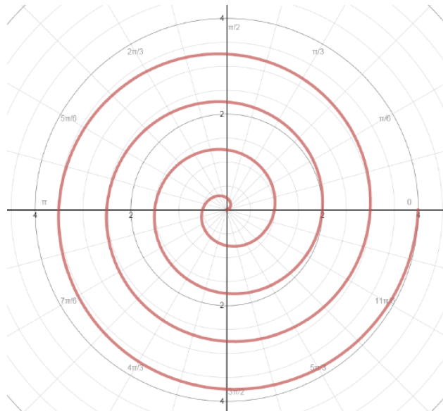
Espiral de Arquímedes r = \theta/2\pi .
