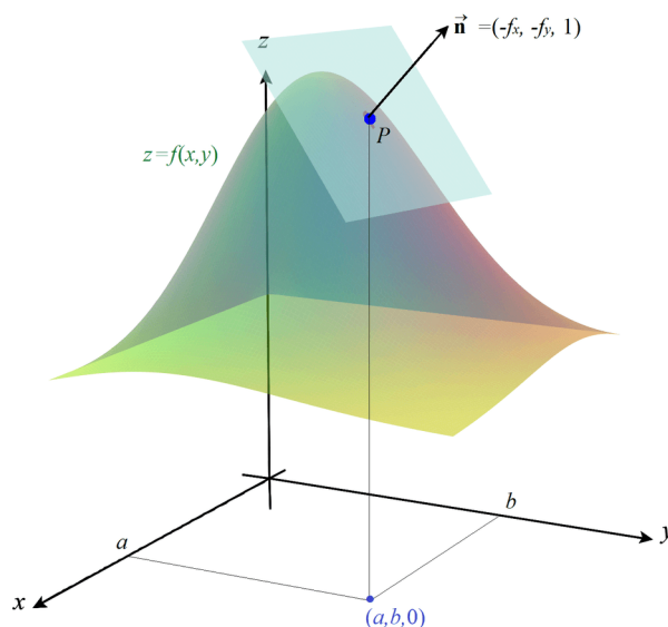
Vector normal y plano tangente.
