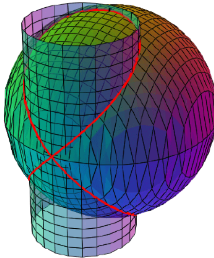
La curva de Viviani.
