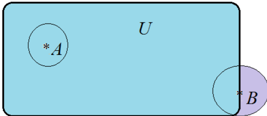
El punto A es un punto interior de U , el punto B está en la frontera de U .
