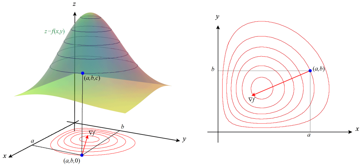
Propiedad de dirección óptima del gradiente.
