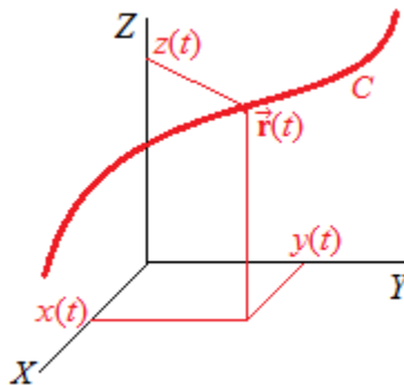
Curva en coordenadas paramétricas.
