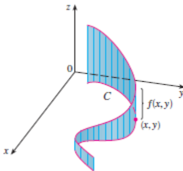
Interpretación geométrica de la integral de línea.
