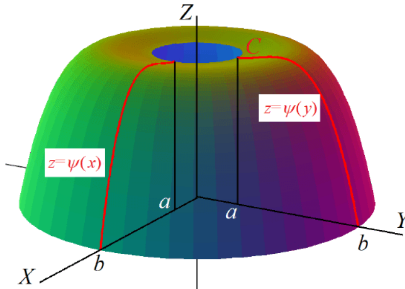
Superficie de revolución alrededor del eje Z .
