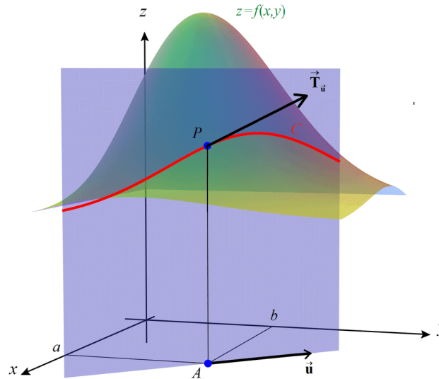
Interpretación geométrica de la derivada direccional.
