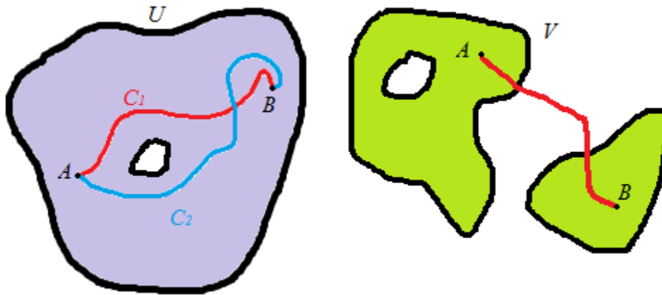
U es conexo. V no es conexo.
