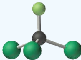
Freon-11, \text{CCl}_3\text{F}
