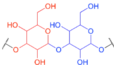
cellulose
