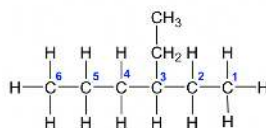
3-ethylhexane
