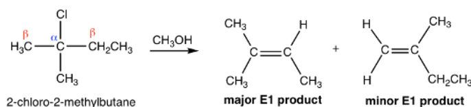
Figure 8.2a Major E1/Minor E1 product
